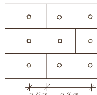
Versetzen der Platten im Verband
