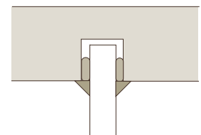
Dichten mit Stopfwohle und Lehmputzmörtel (auf dem Holz ggf. mit Putzträger)
