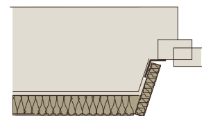
Luftdichtung und Dämmung in der Fensterleibung
